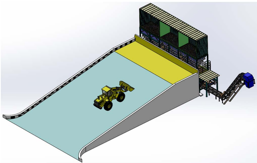
主方案：斜坡铲车上料
