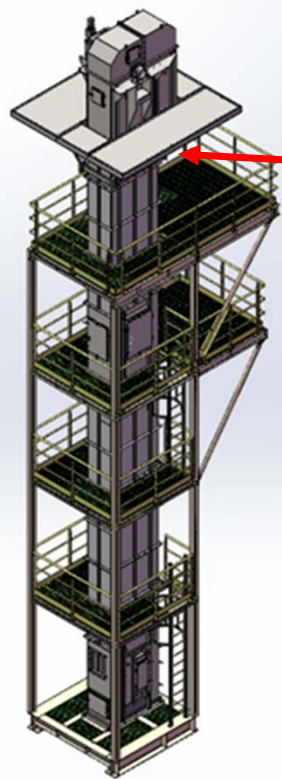
喂料楼模块
