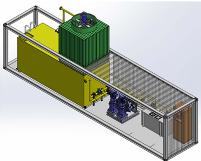
水 stations 模块
