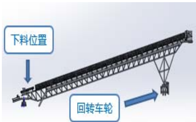
备选方案二：回转上料
