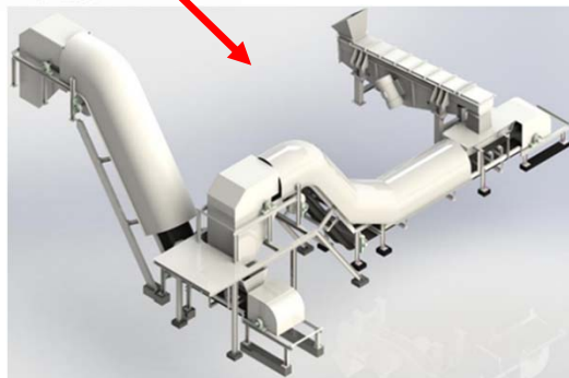
磨机回料模块
