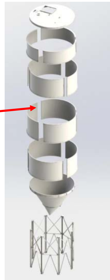
水泥库模块
