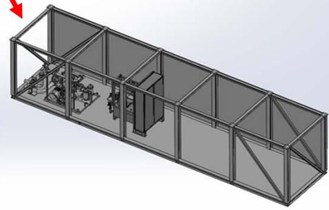
磨机润滑、液压系统模块
